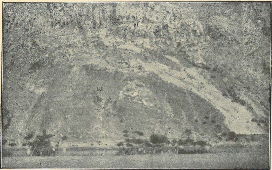
Fig. 1. Untere ( Ut ) und obere ( ot ) Trias des Jubani bei Vau Denjs.
