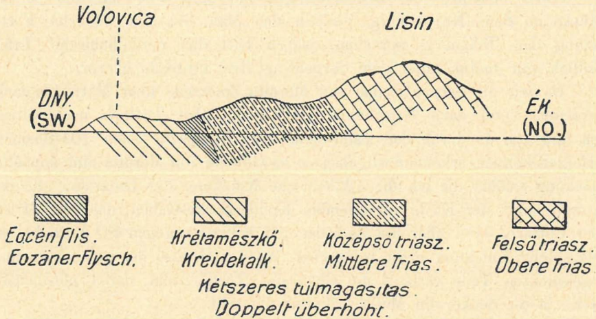
Fig. 4. Profil des Lisin in Montenegro (nach MARTELLI).
