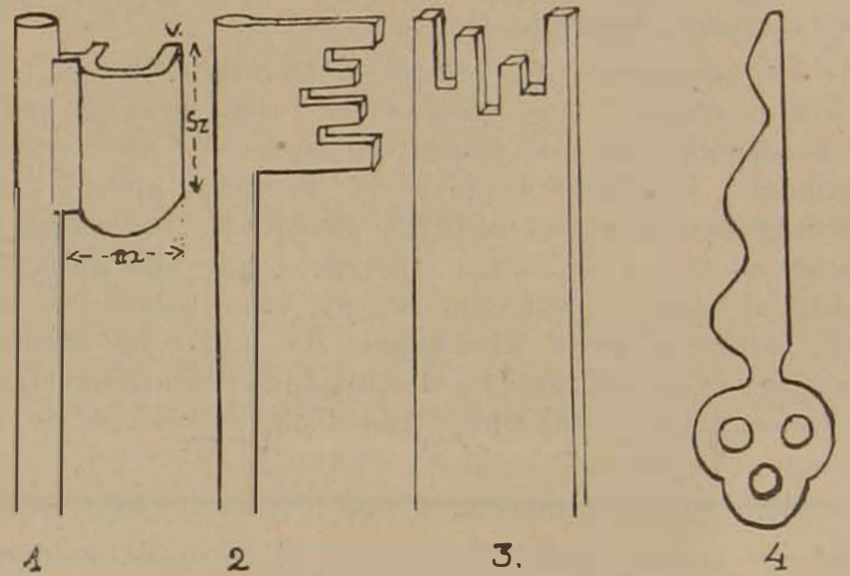
1. - egyszerű zár kulcstolla 3. - biztonság (Brahma-zár) kulcstolla 2. - biztonság (Chubb-zár) kulcstolla 4. - Yale-zár kulcstolla m - a kulcstoll magassága, Sz - szélessége v - vastagsága
