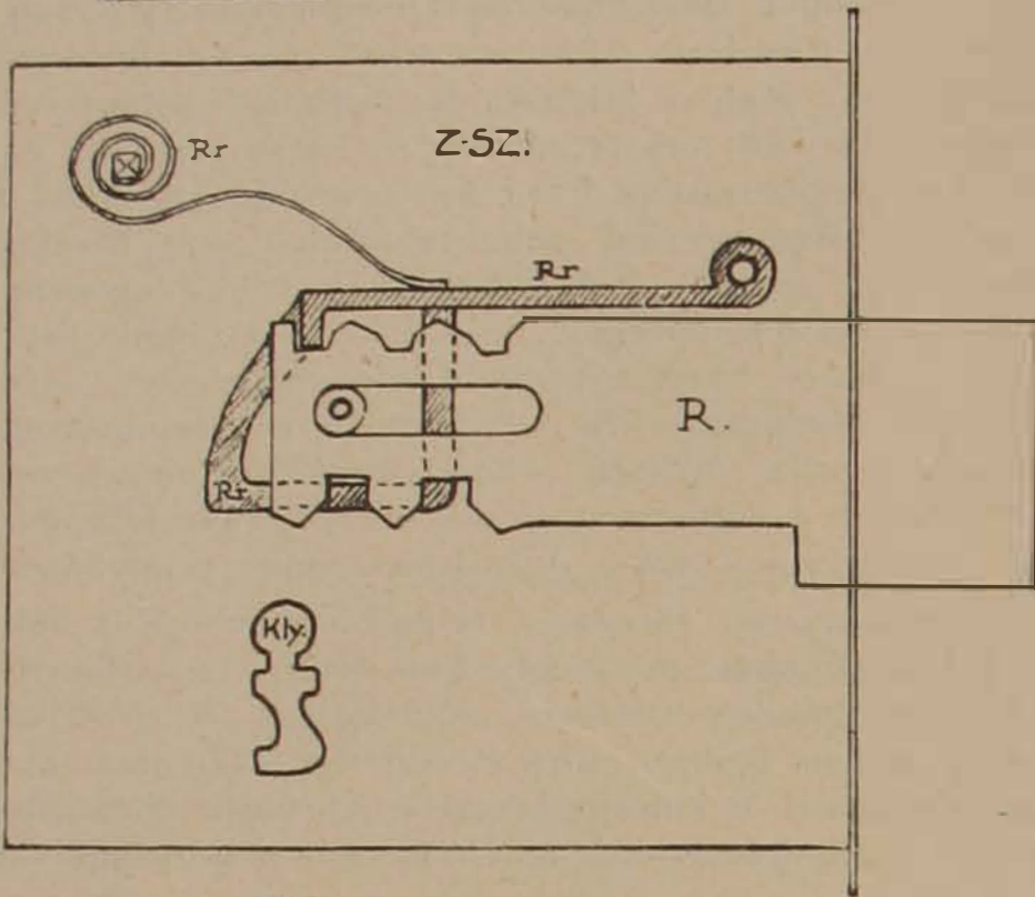
Z-SZ. - zártekercsény Rr. - reteszrugó R. - retesz Kly. - kulcslyuk
