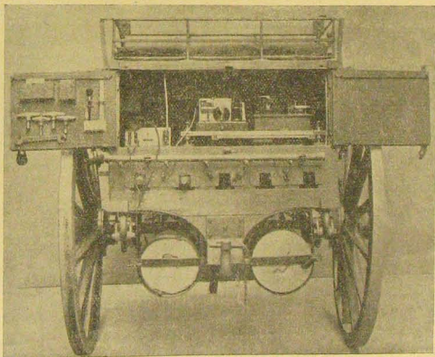
A német hadsereg drótnélküli táviró-berendezése. Leadó szerkezet.
