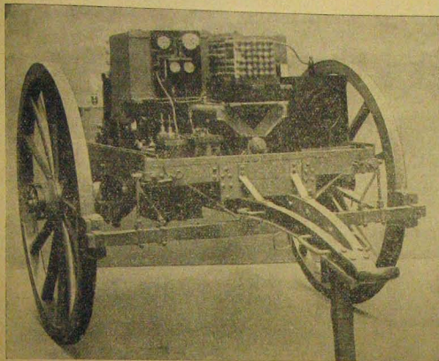
A német hadsereg drótnélküli táviró-berendezése. Feladó szerkezet.
