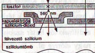
8. ábra. Fent: normál- és vékony, lent: UV konverteres CCD
