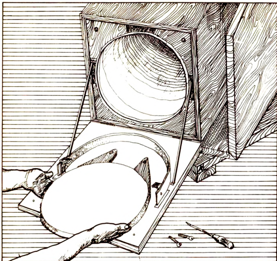
3. ábra. A tükör befogása Dobson-szerelésnél.
