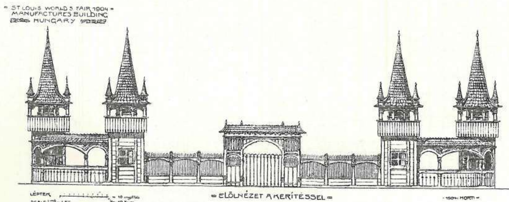
A ST. LOUISI VILÁGKIÁLLÍTÁS IPARCSARNOKÁBAN LEVŐ MAGYAR OSZTÁLYNAK KERITÉSE. TERVEZTE HORTI PÁL.
